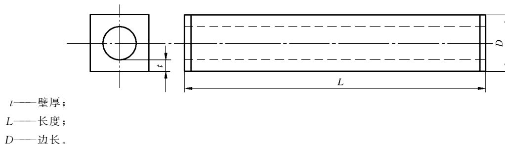
图 1 空心方桩的图示
